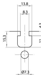
Cava 8 mm (serie 45) 8 mm slot (series 45)
