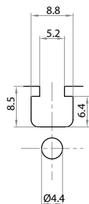
Cava 5 mm 5 mm slot
