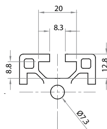
Cava 8 mm (serie 40) 8 mm slot (series 40)
